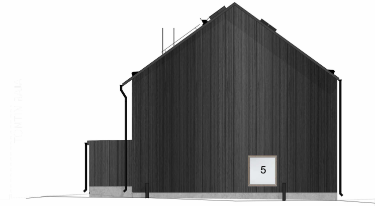
Julkisivu länteen
