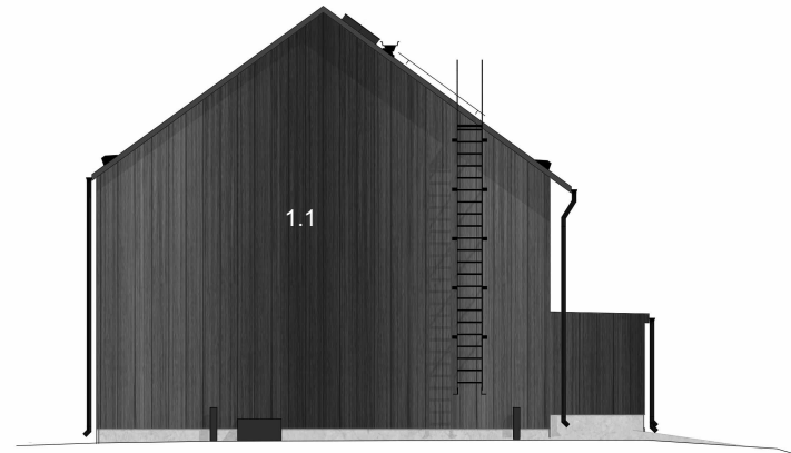
Julkisivu itään
