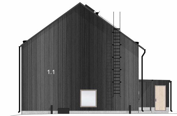
Julkisivu itään
