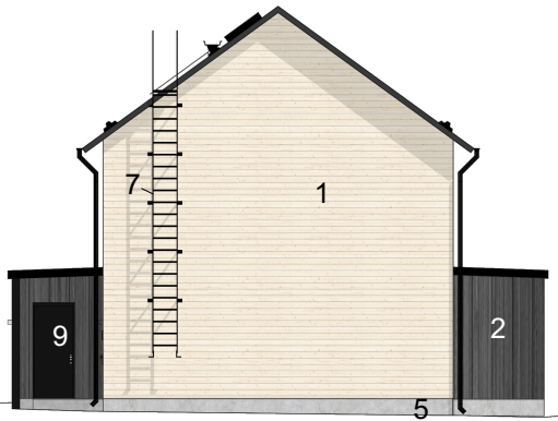
JULKISIVU LUOTEESEEN
