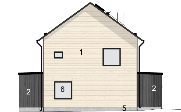
JULKISIVU LUOTEESEEN
