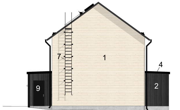
JULKISIVU KAAKKOON
