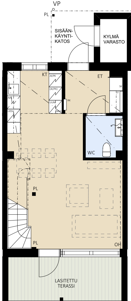
1. KERROS
